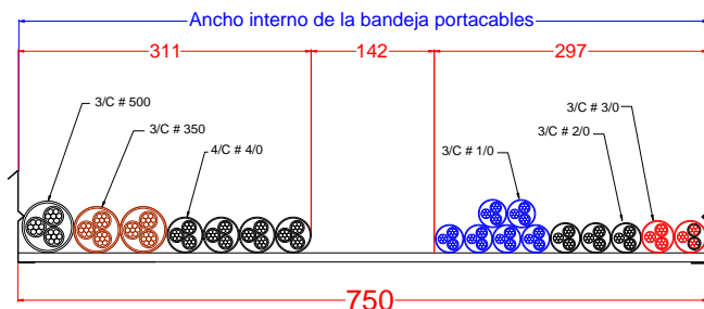
Cables menores y mayores a 4/0 AWG colocados en la bandeja portacables Figura 3
