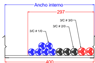
Cables mayores o iguales al calibre 4/0 AWG Figura 2
