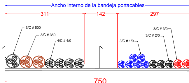
Barrera divisora Figura 4
