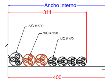
Cables mayores o iguales al calibre 4/0 AWG
